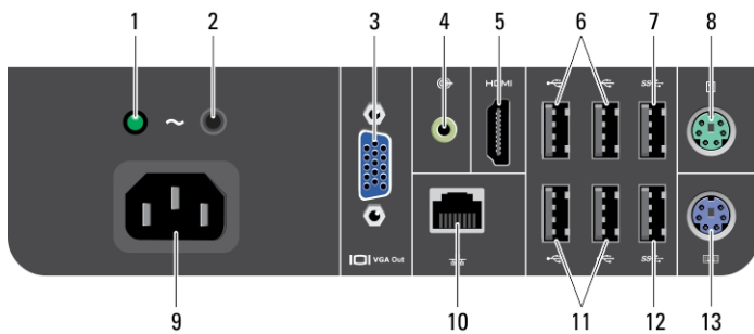
圖 3. 背面板視圖
